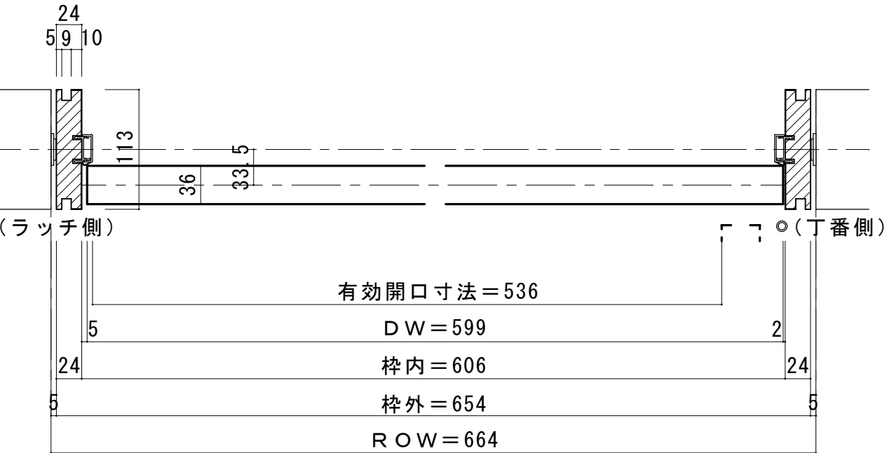
■横断面図
