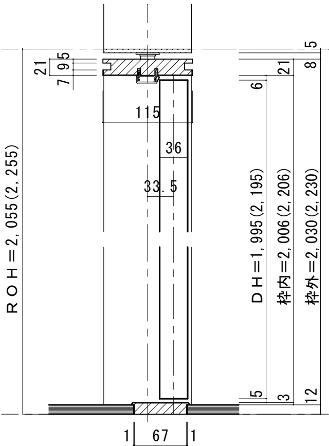
■縦断面図
