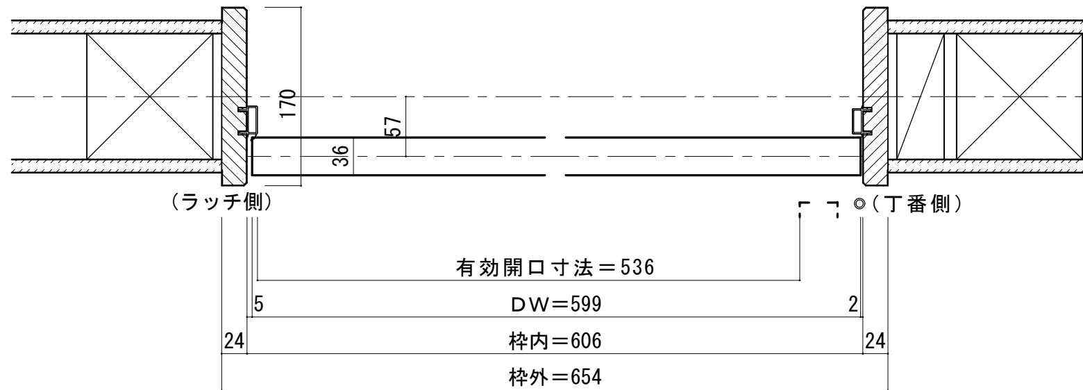
■横断面図
