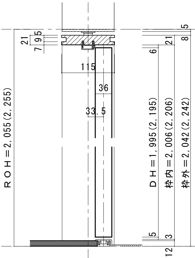
■ 縦断面図 [片ツハタイプ]
