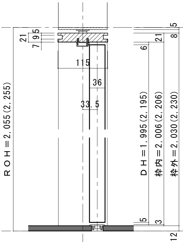
■ 縦断面図 [両ツハタイプ]
