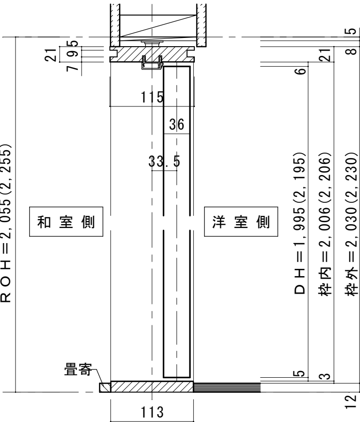
■縦断面図
