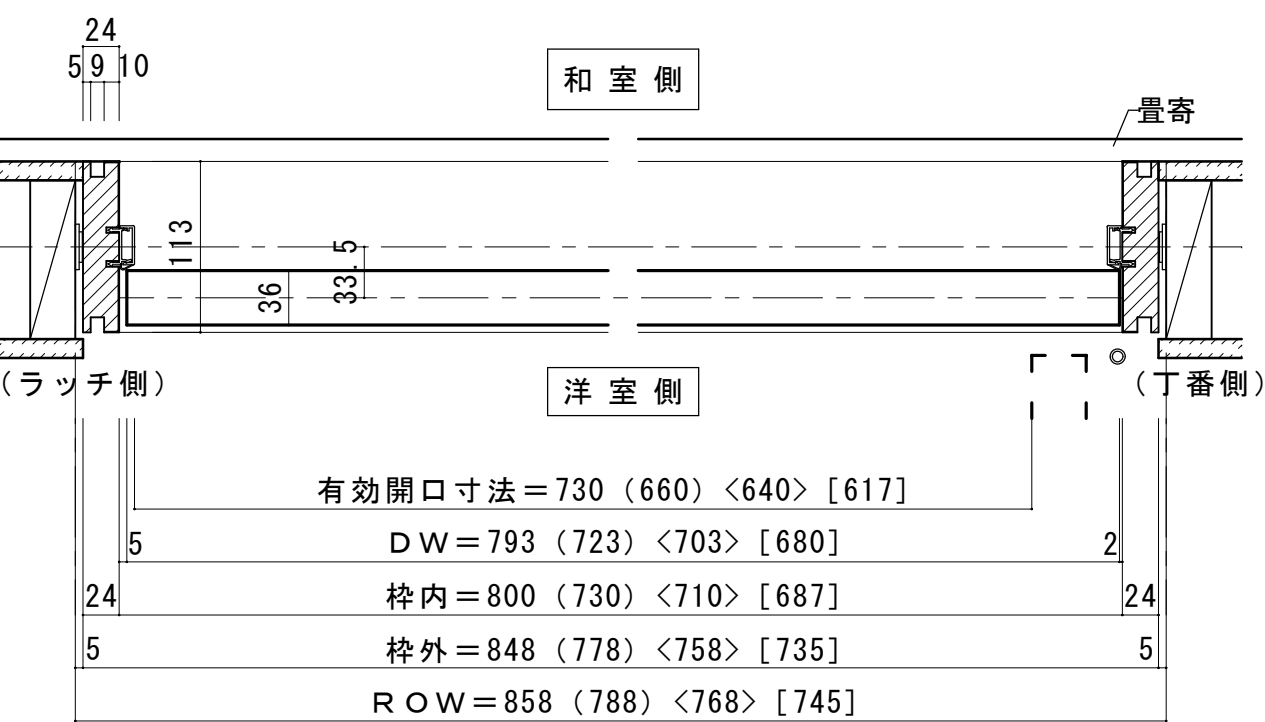
■横断面図
