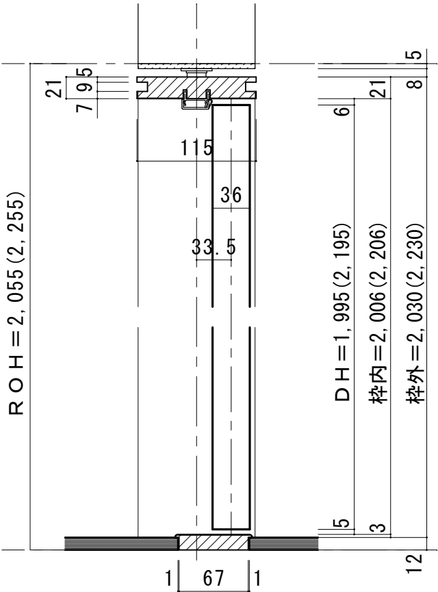
■ 縦断面図
