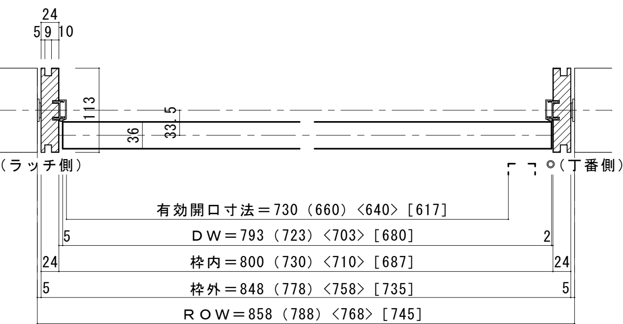
■ 横断面図
