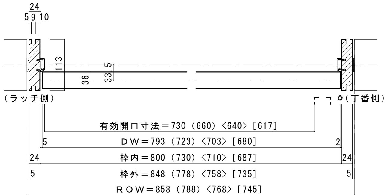
■ 横断面図
