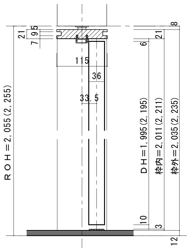
■ 縦断面図
