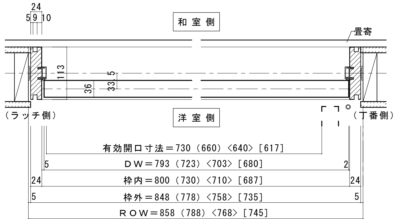
■横断面図
