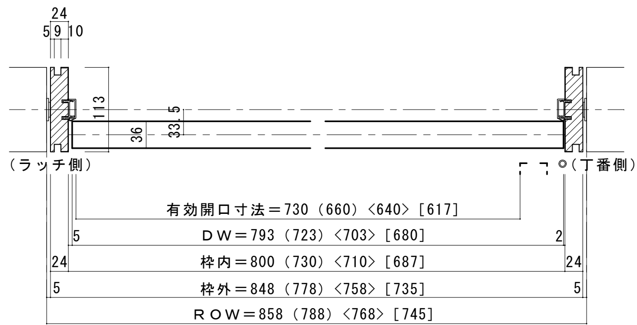
■ 横断面図
