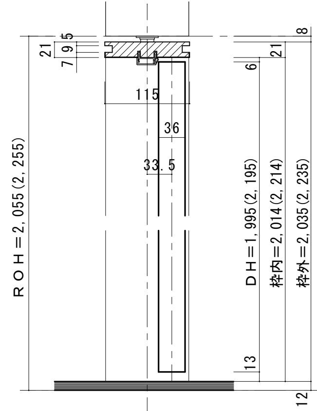
■ 縦断面図
