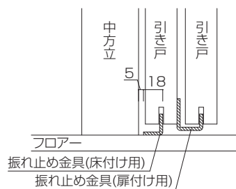
2枚引き込み戸の場合
