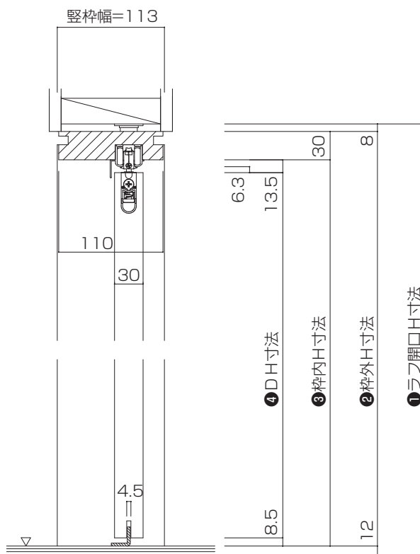
縦断面図
