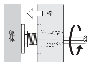
枠を外側に出す場合
