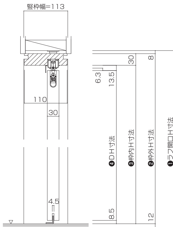
縦断面図
