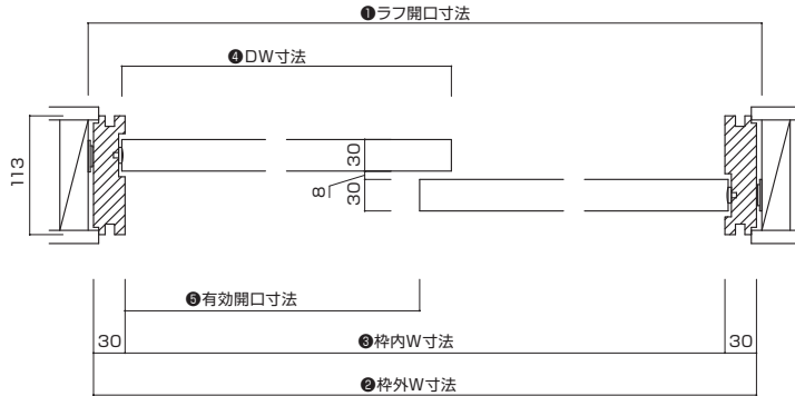
横断面図
