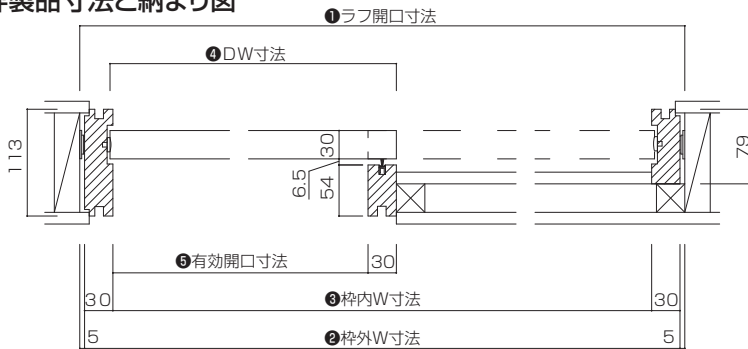
横断面図
