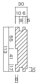
豎杵(開口部側)
