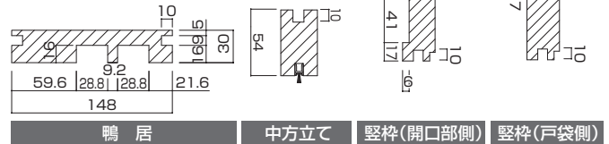
縦断面図
