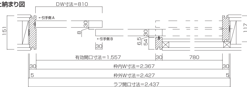
横断面図
