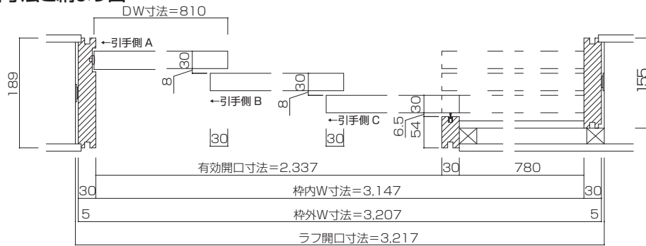
横断面図
