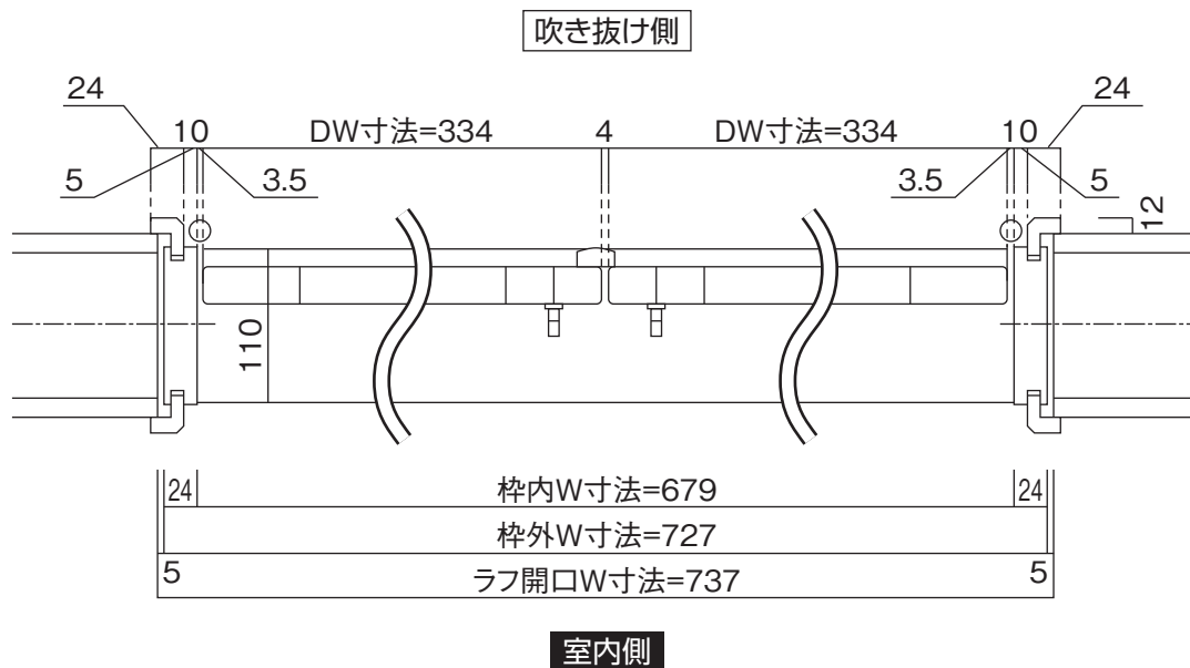
横断面図
