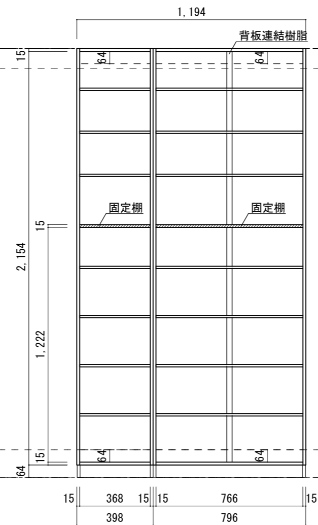
キャビネット図
