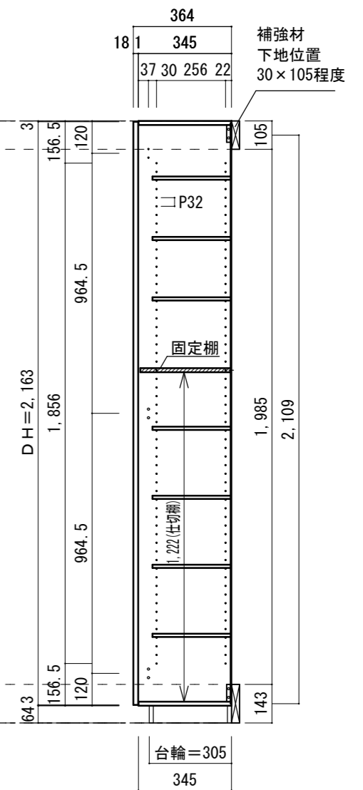
A-A' 断面図
