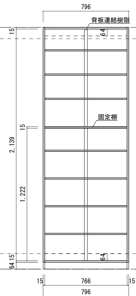
キャビネット図
