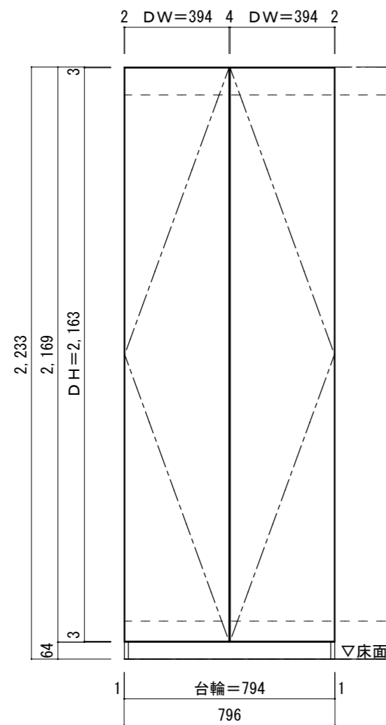
扉配置図
