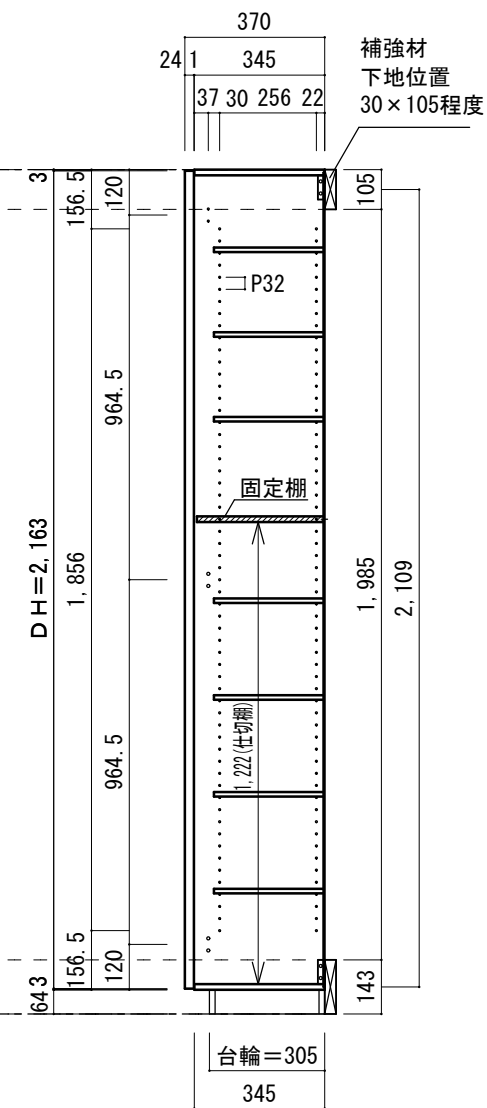
A-A' 断面図
