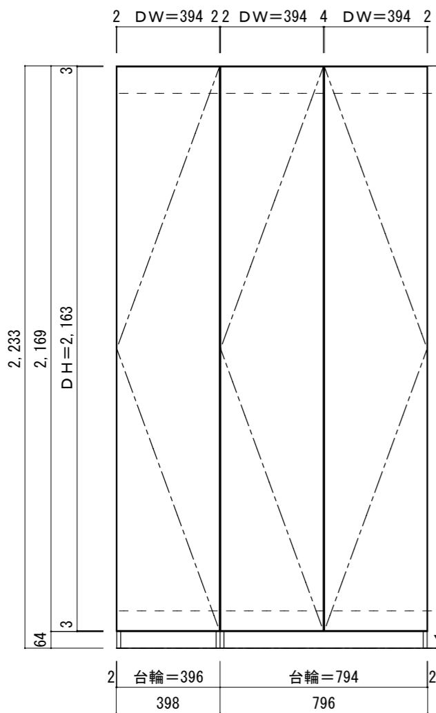
扉配置図
