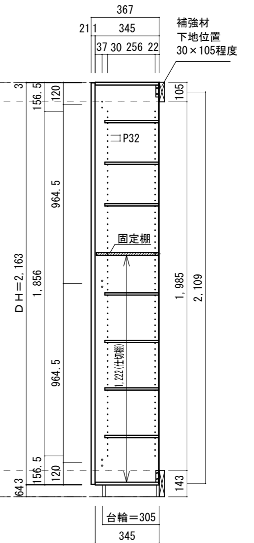
A-A' 断面図
