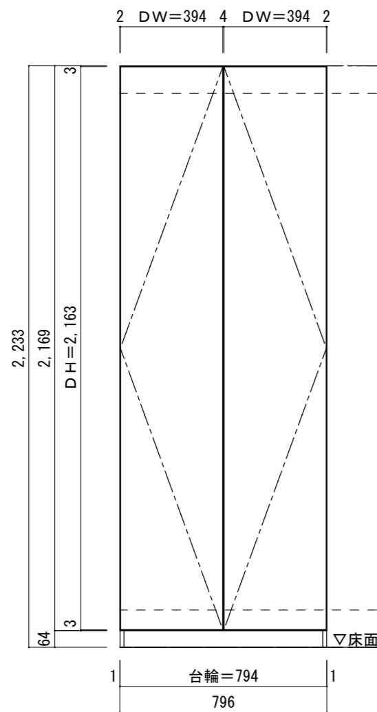
扉配置図
