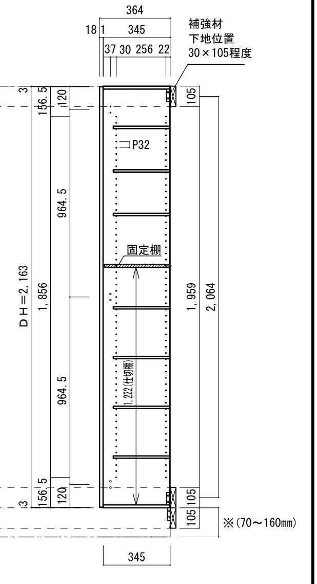
A-A' 断面図
