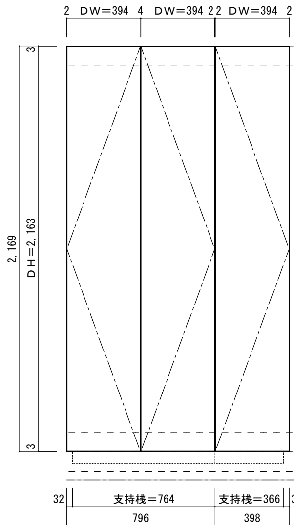
扉配置図
