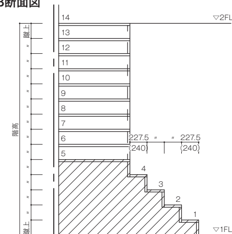
B-B断面図
