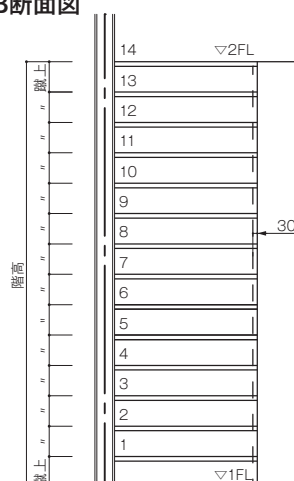
B-B断面図
