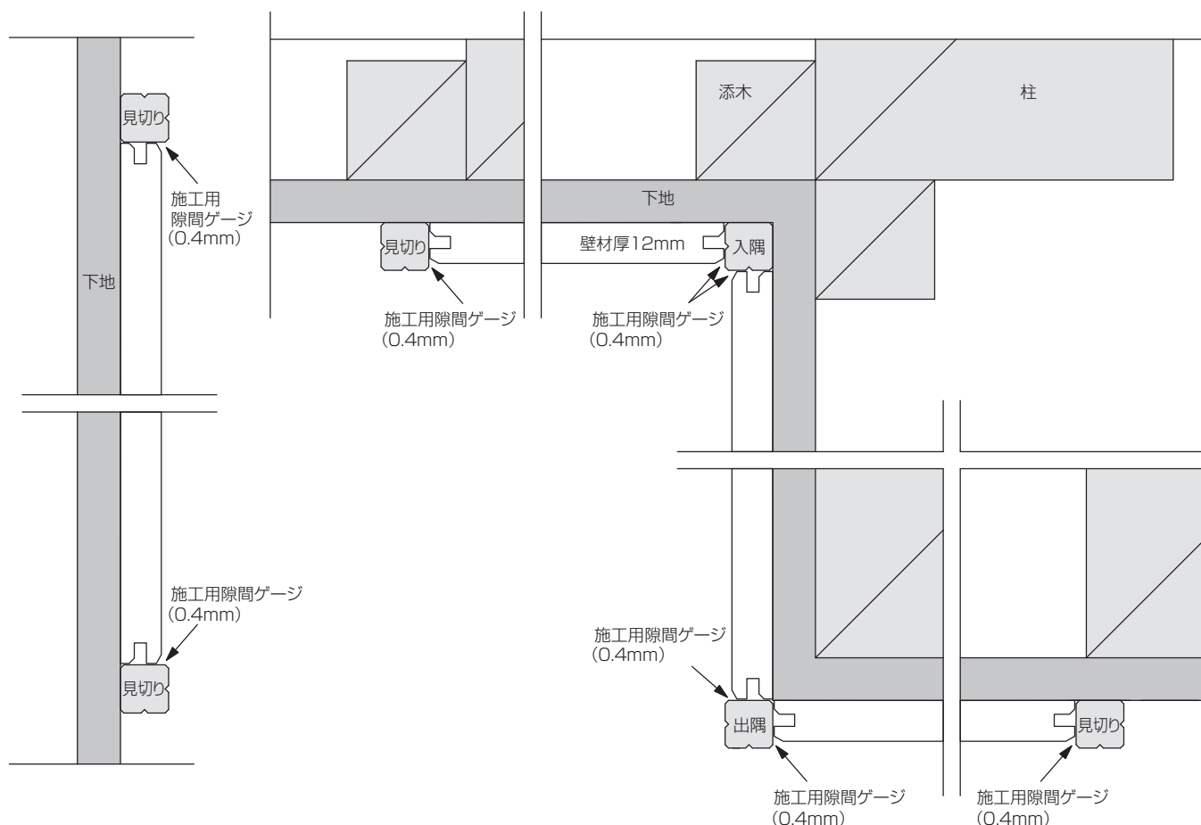
使用側面図
