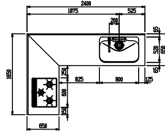
(W2400×W1650)
