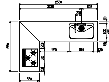
(W2550×W1650)
