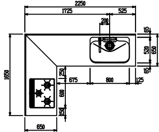
(W2250×W1650)
