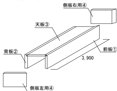
■組立全体図 S=1/10
