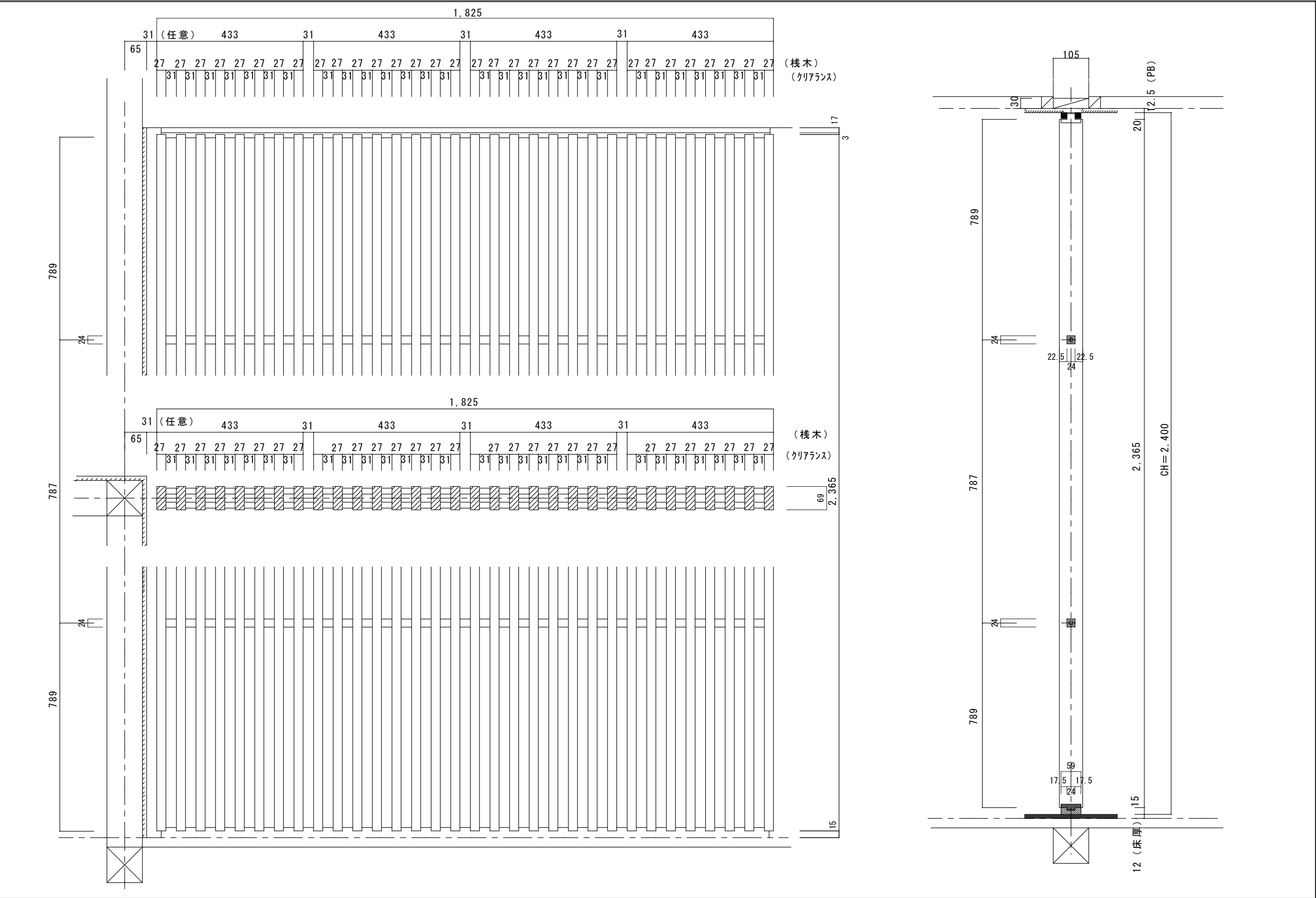
ジュピーノ・J たて格子スクリーンパネル 4セットの場合
