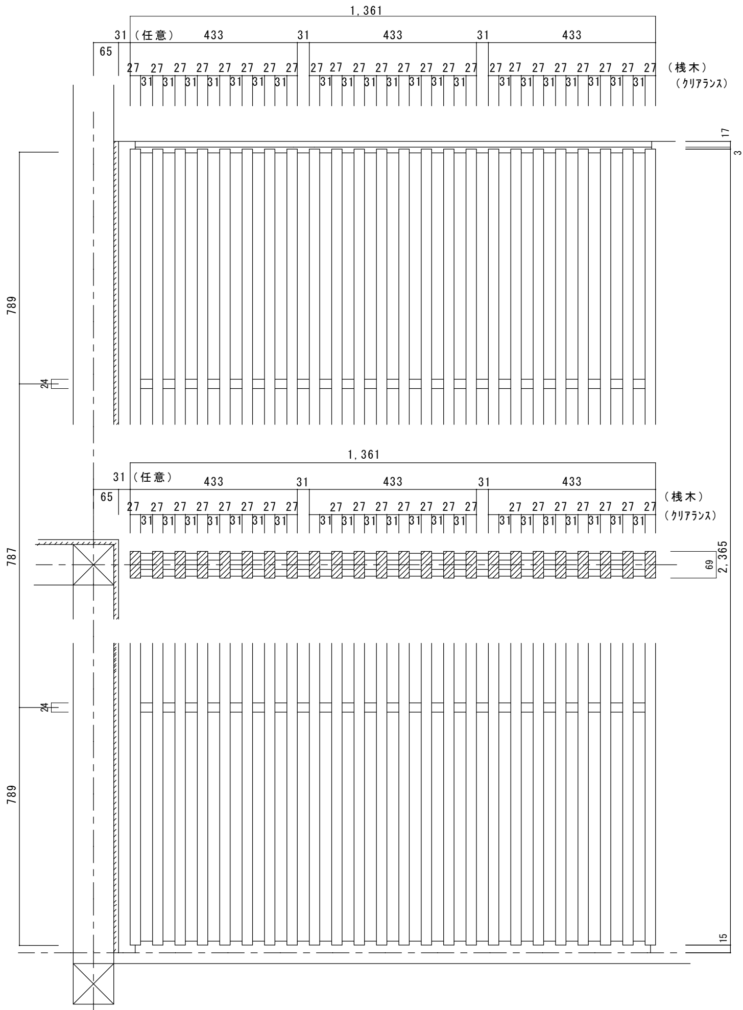
図面名 JUPINO・J 格子スクリーン納まり図
