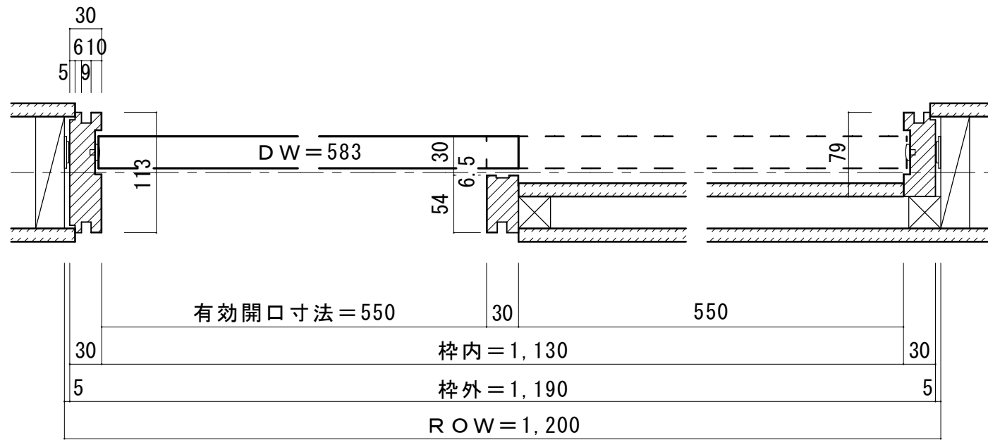
■横断面図
