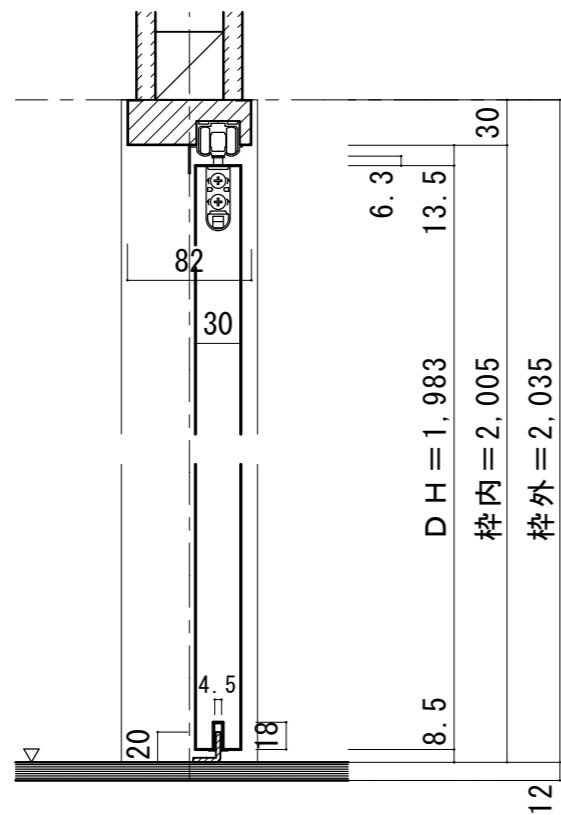
■縦断面図
