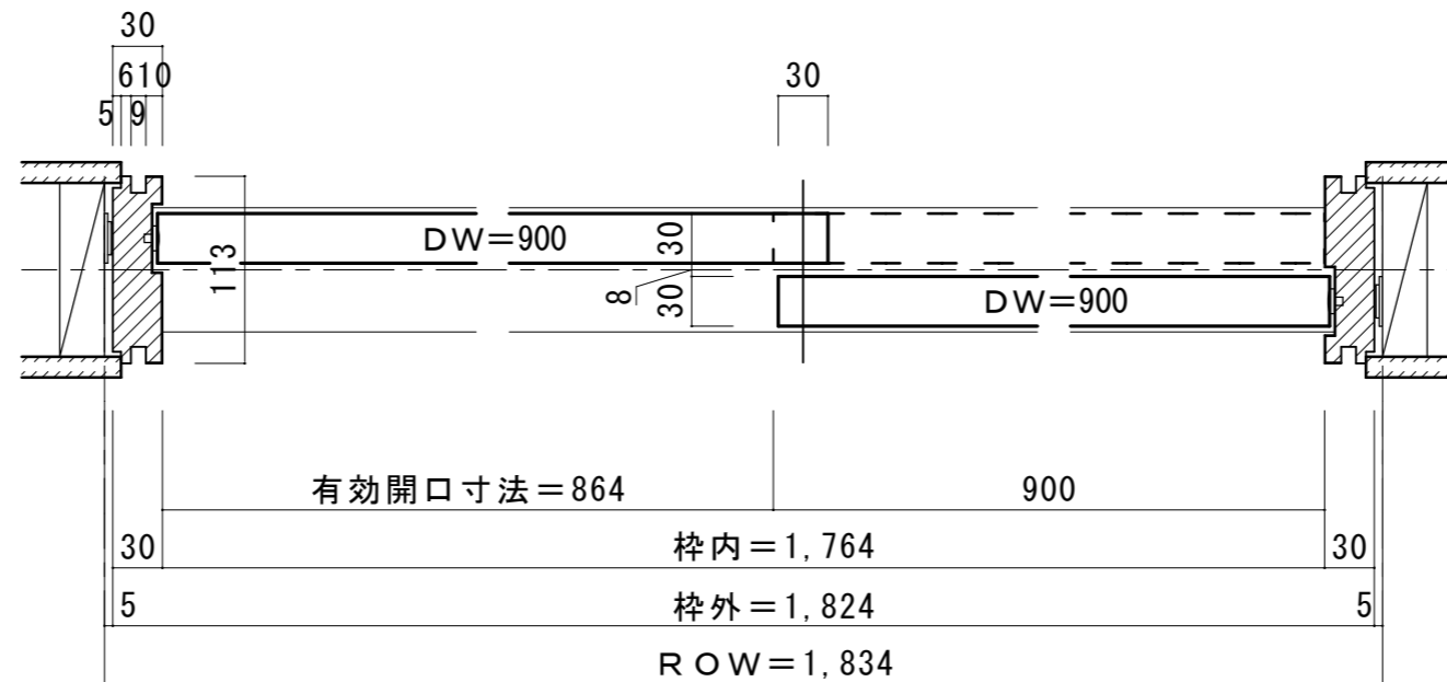
■横断面図
