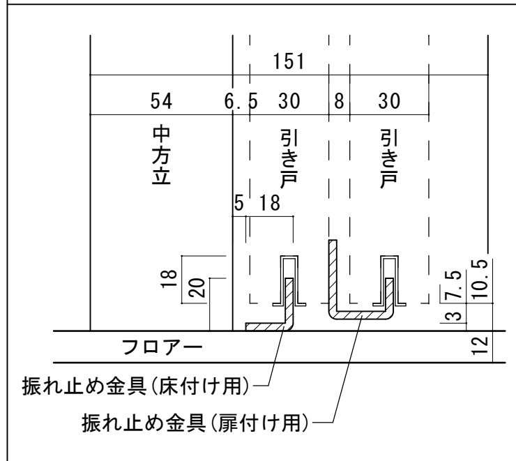
振れ止め金具取り付け位置 (S=1/2)
