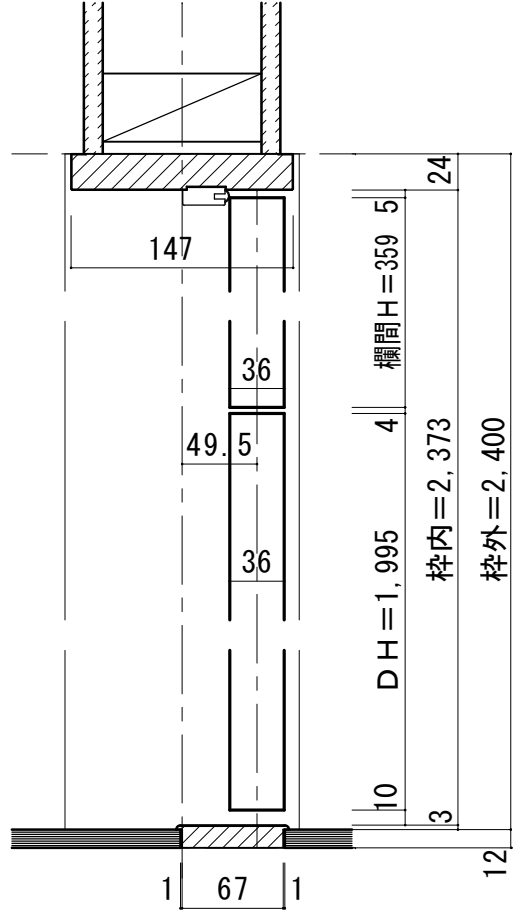
■ 縦断面図[4方枠]
