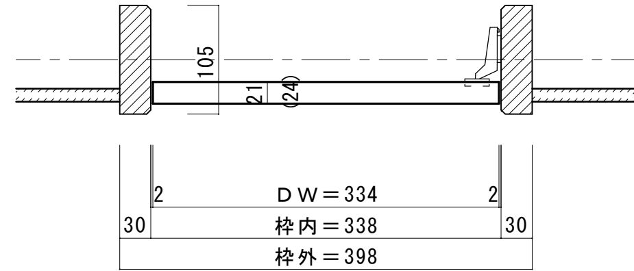
■横断面図 H=4尺、3尺
