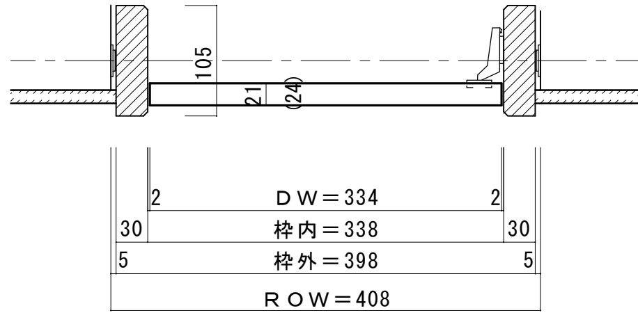
■横断面図 H=8尺、7尺、6尺
