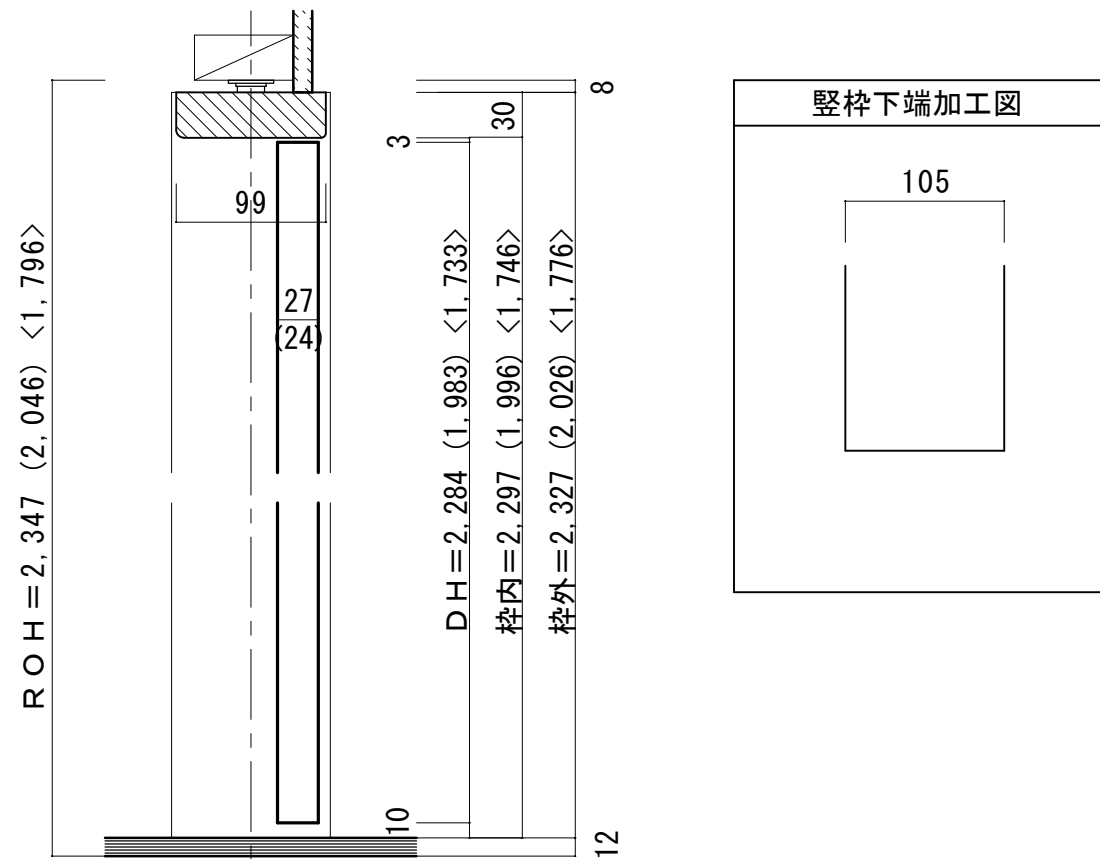
■縦断面図 H=8尺（7尺）〈6尺〉
