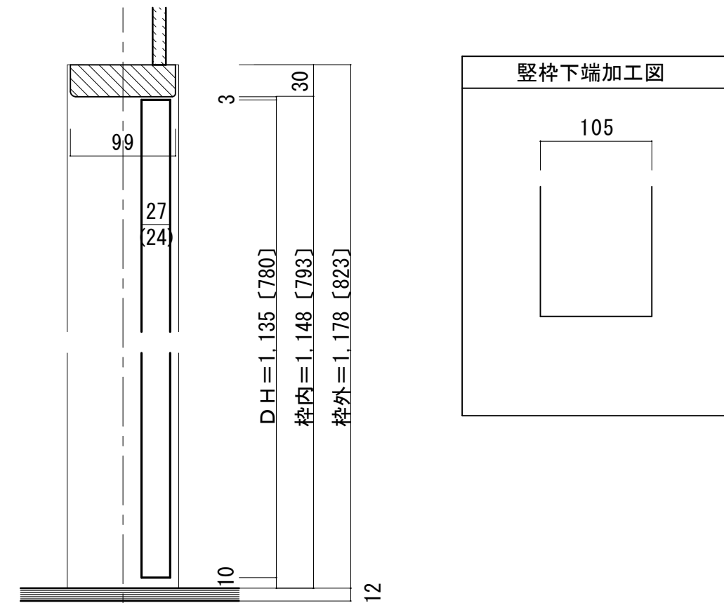
■縦断面図 H=4尺〔3尺〕
