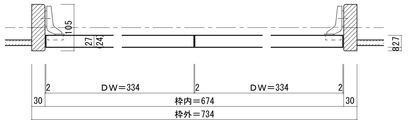
■横断面図 H=4尺、3尺
