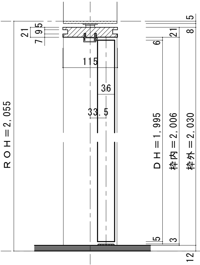
■ 縦断面図
