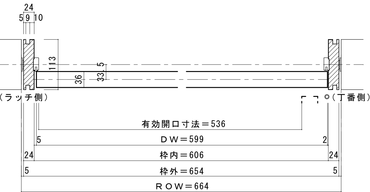
■ 横断面図
