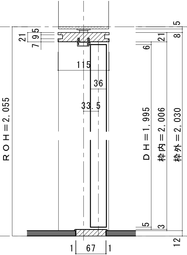
■縦断面図
