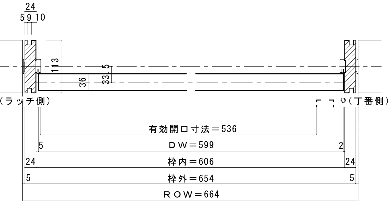
■横断面図
