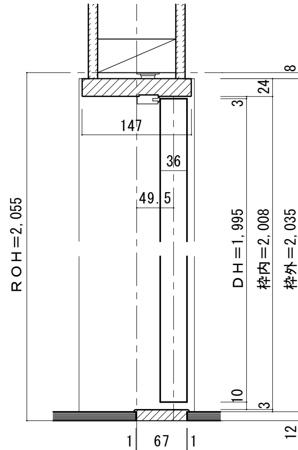
■縦断面図
