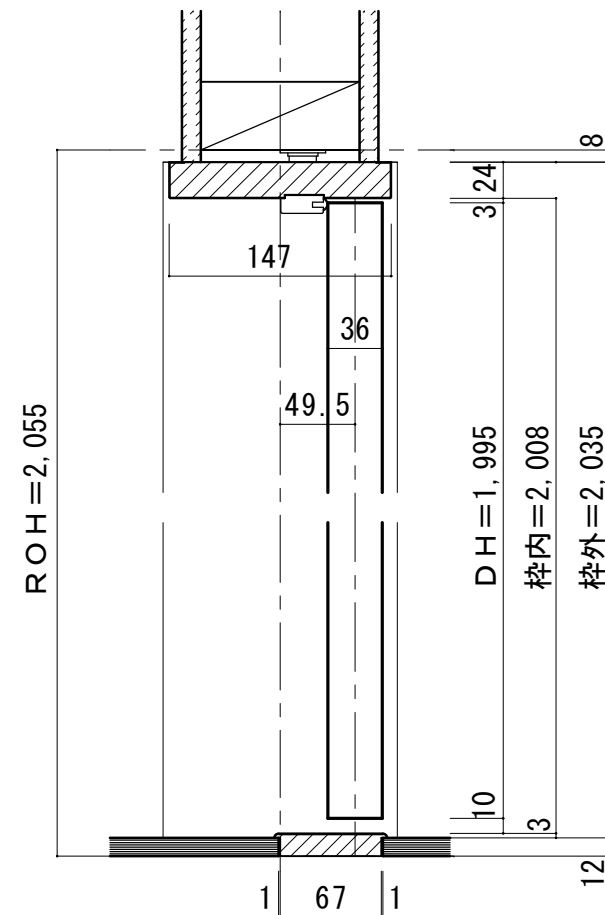
■縦断面図
