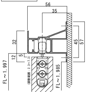
レール取付高さ
