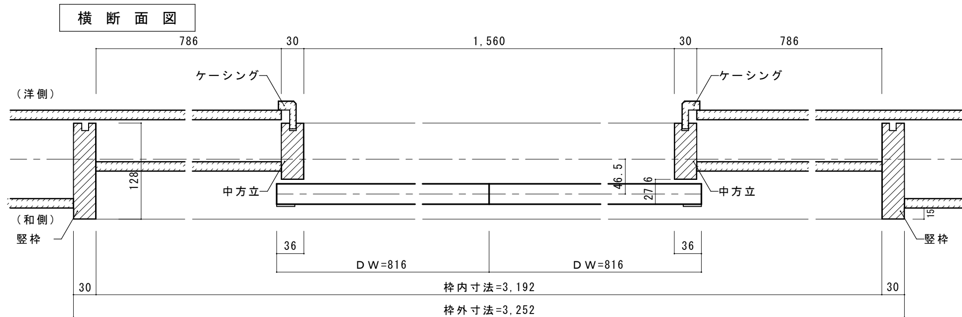
■ ケーシング寸法図
