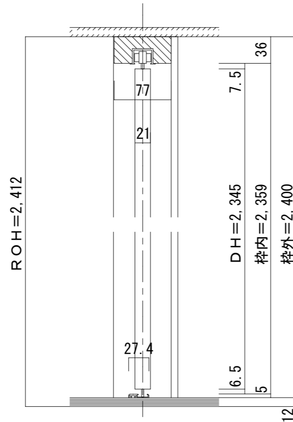
■縦断面図
