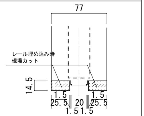
■ 縦枠下端加工図 (S=1/3)
