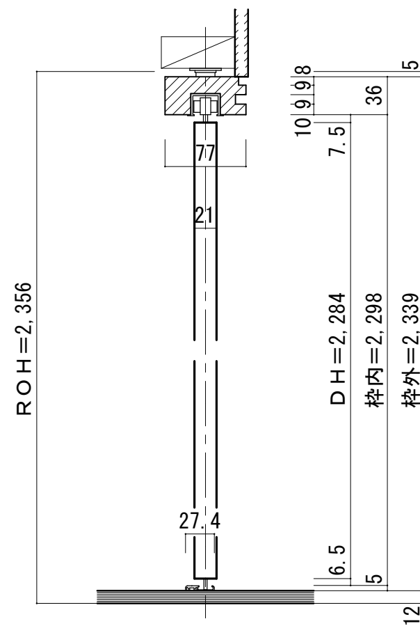
■縦断面図
