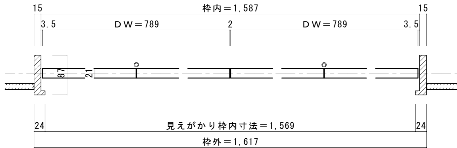
■横断面図[間口6尺]
