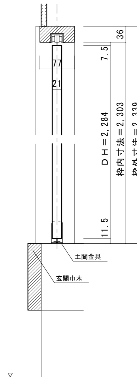
■縦断面図
