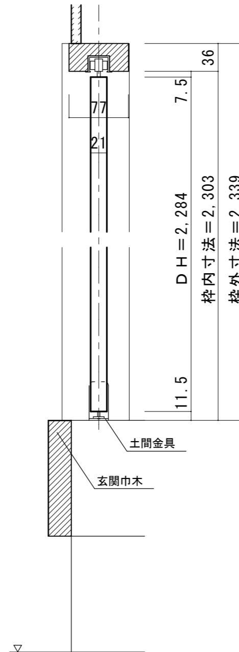
■縦断面図
