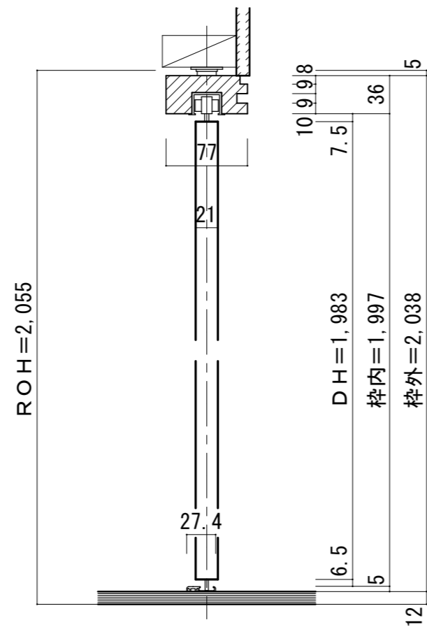
■縦断面図
