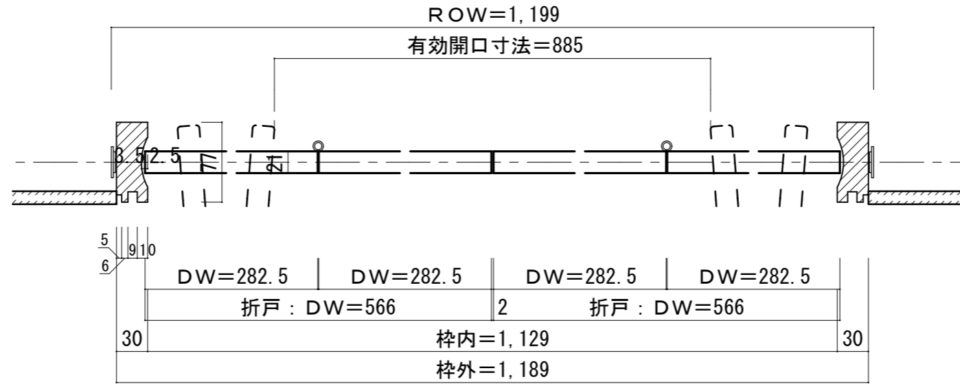
■横断面図
