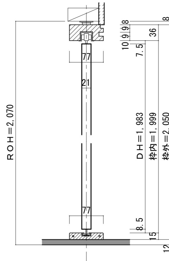
■縦断面図
