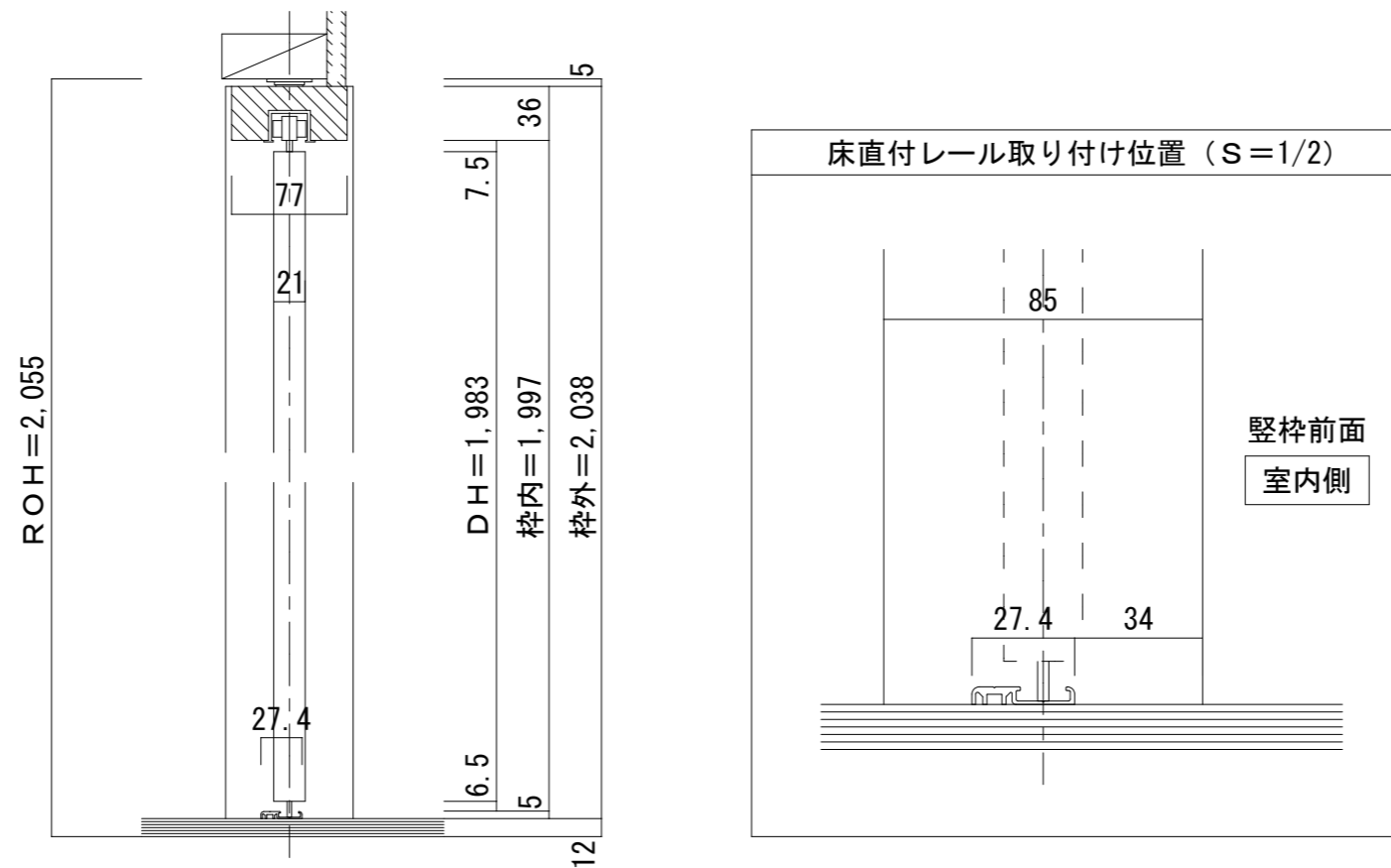
■縦断面図
