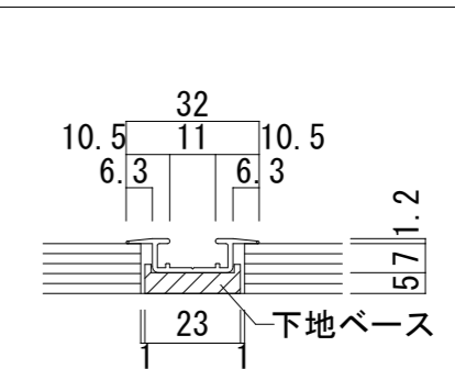
■ レール拡大図 (S=1/2)
