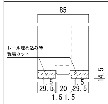
■ レール拡大図 (S=1/2)
